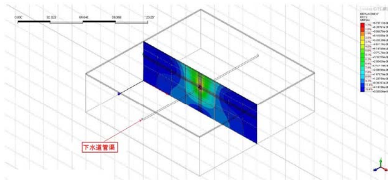
地盤変位コンター④
