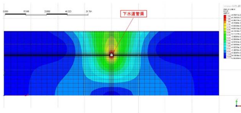
地盤変位コンター④
