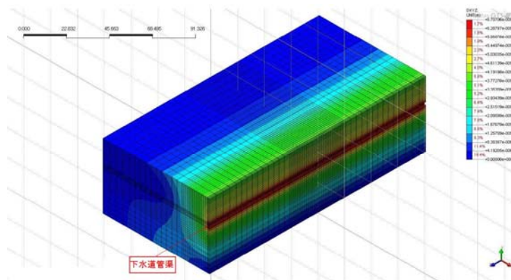
地盤変位コンター③0図
