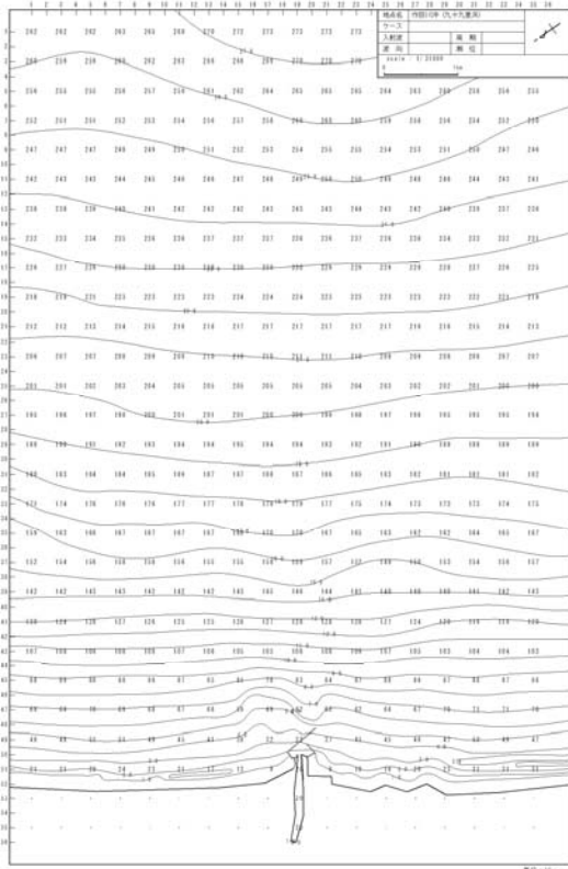
図一 水深分布図
