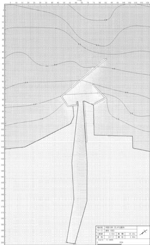
図一 波向ベクトル分布図（入射波）
