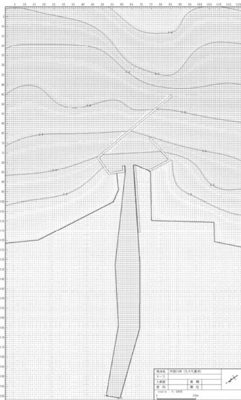
図一 水深分布図
